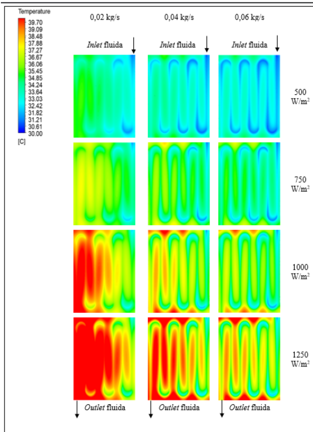
GAMBAR 10. Hasil simulasi pendinginan permukaan bawah.
