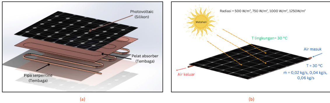
GAMBAR 3. (Parameter pendinginan permukaan bawah (a) susunan material pendinginan bawah, (b) kondisi batas pendinginan permukaan bawah.
