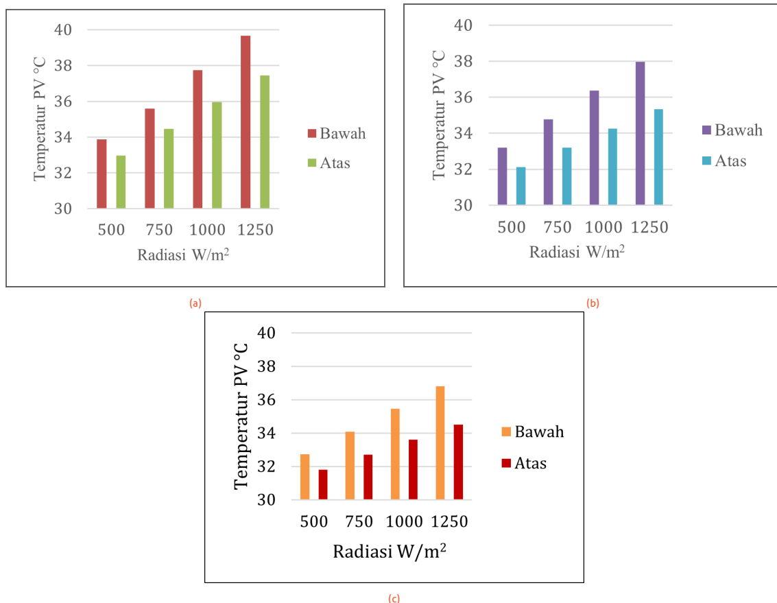
GAMBAR 11. Grafik temperatur permukaan Photovoltaic terhadap radiasi untuk berbagai metode pendinginan dan laju aliran massa (a) 0,02 kg/s, (b) 0,04 kg/s, (c) 0,06 kg/s.
