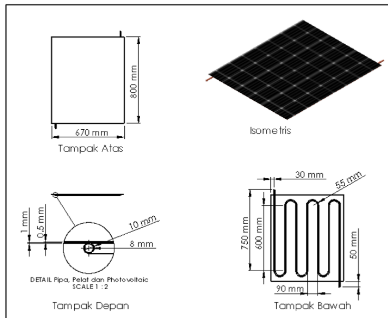
GAMBAR 1. Geometri kolektor Photovoltaic/Thermal dengan pelat absorber dan pipa serpentine .
