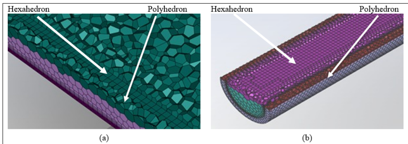
GAMBAR 4. (a) Meshing pendinginan permukaan atas, (b) Meshing pendinginan permukaan bawah.
