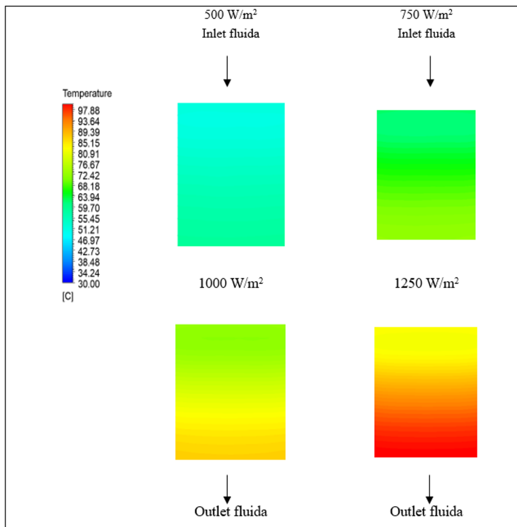
GAMBAR 8. Hasil simulasi permukaan Photovoltaic berdasarkan pendinginan alami.
