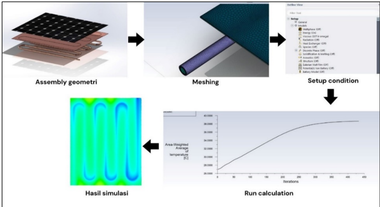
GAMBAR 5. Langkah-langkah simulasi Computational Fluid Dynamic .
