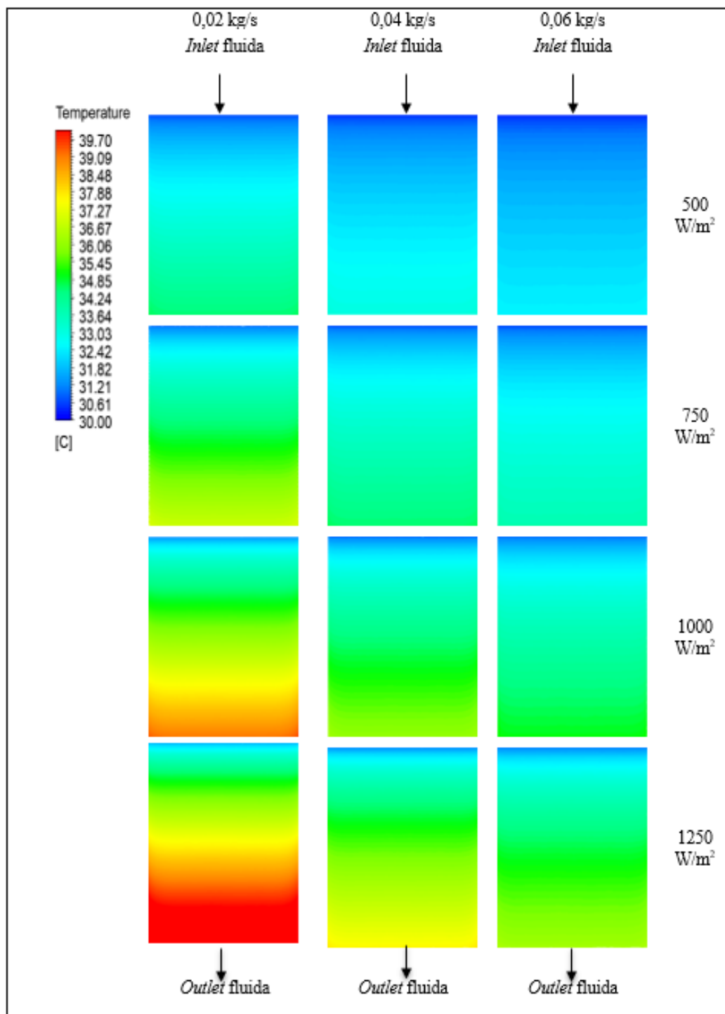
GAMBAR 9. Hasil simulasi pendinginan permukaan atas.
