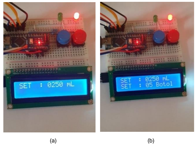
Gambar 5. Proses memasukkan nilai, (a) takaran volume, (b) jumlah botol.
