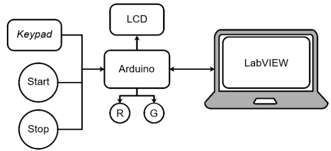
Gambar 1. Diagram blok sistem mesin pengisian cairan otomatis.
