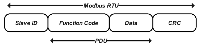
Gambar 4. Pesan Modbus RTU.
