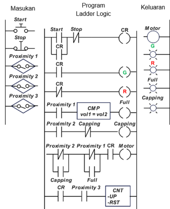
Gambar 2. Ladder logic pada sistem mesin pengisian cairan otomatis.
