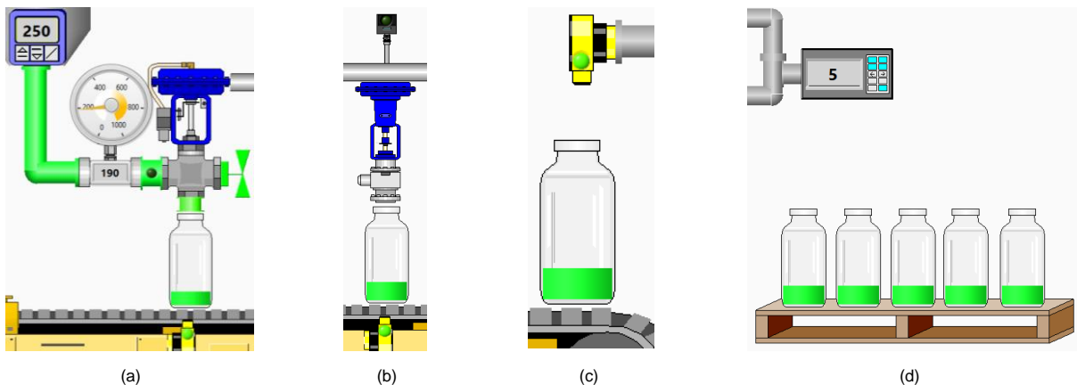
Gambar 7. Proses hasil simulasi pada front panel LabVIEW, (a) pengisian, (b) penutupan, (c) penghitungan, (d) jumlah botol.
