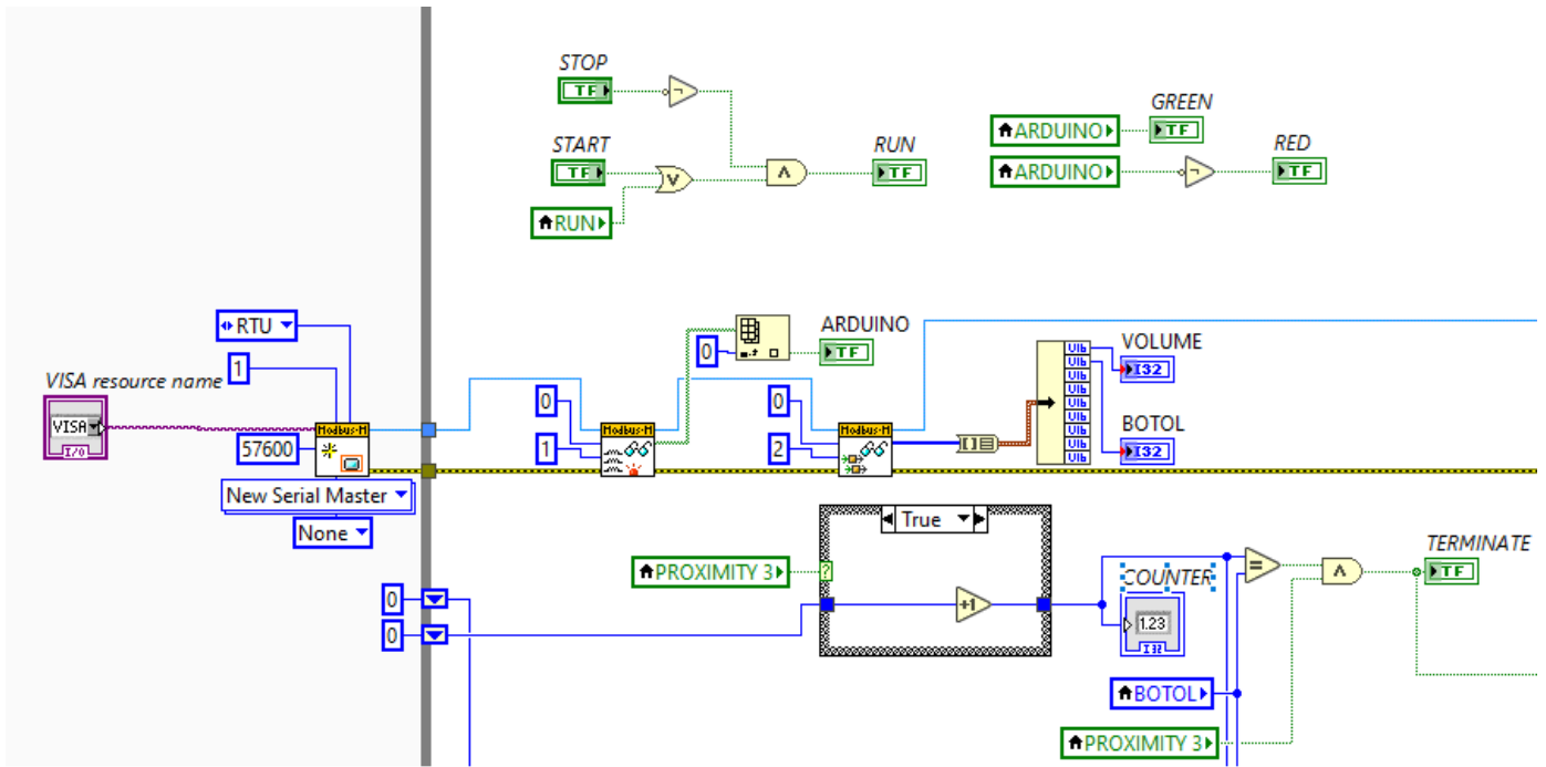
Gambar 6. Diagram blok Modbus pada LabVIEW.
