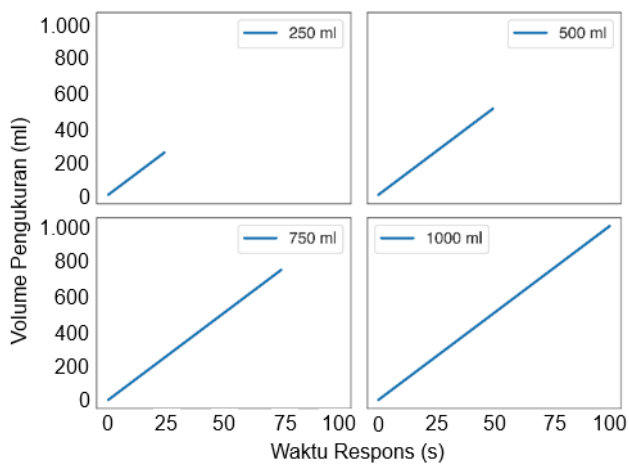
Gambar 8. Waktu respons terhadap takaran volume.
