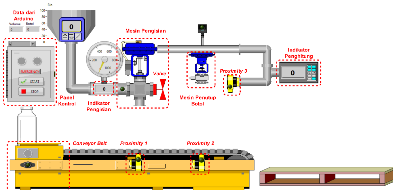
Gambar 3. Komponen sistem mesin pengisian cairan otomatis pada front panel LabVIEW.
