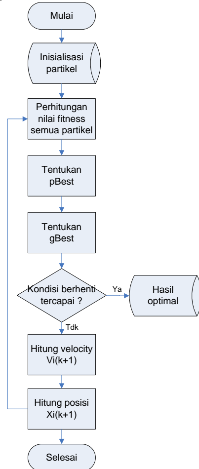
Gbr. 1 Diagram alir PSO
