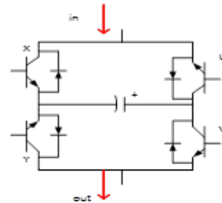
Gbr. 2 Rangkaian ketika menggunakan MERS untuk memperbaiki daya motor induksi.
