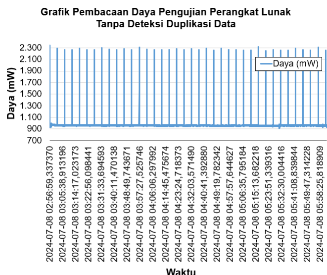
Gambar 4. Grafik pembacaan daya pengujian perangkat lunak tanpa deteksi duplikasi data.
