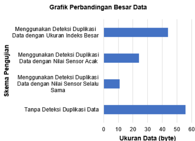
Gambar 10. Perbandingan ukuran data yang dikirimkan oleh perangkat lunak tanpa penggunaan deteksi duplikasi data dan perangkat lunak dengan penggunaan deteksi duplikasi data.
