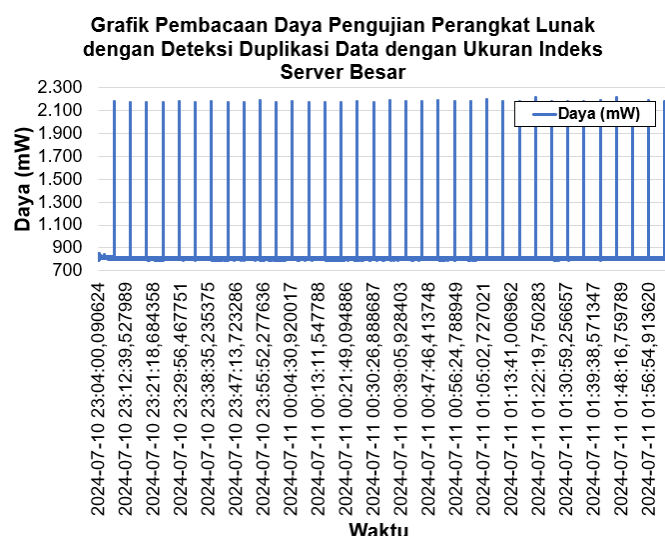
Gambar 7. Grafik hasil pembacaan daya pengujian perangkat lunak menggunakan deteksi duplikasi data dengan data indeks server berukuran besar.
