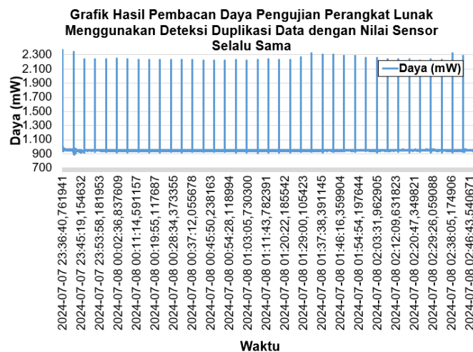
Gambar 5. Grafik hasil pembacaan daya pengujian perangkat lunak menggunakan deteksi duplikasi data dengan data pembacaan sensor selalu sama.
