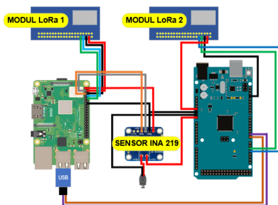
Gambar 3. Skematik pengujian perangkat lunak.
