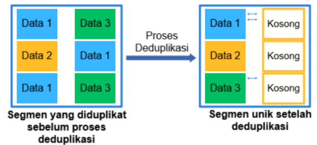
Gambar 1. Proses deteksi duplikasi data.
