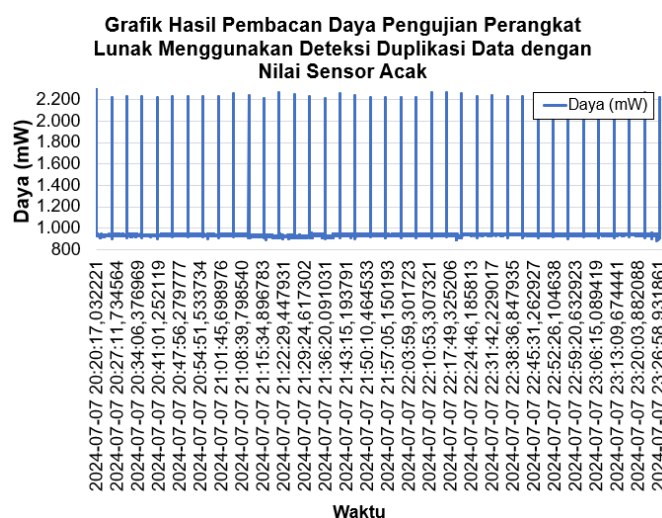
Gambar 6. Grafik hasil pembacaan daya pengujian perangkat lunak menggunakan deteksi duplikasi data dengan data pembacaan sensor acak.
