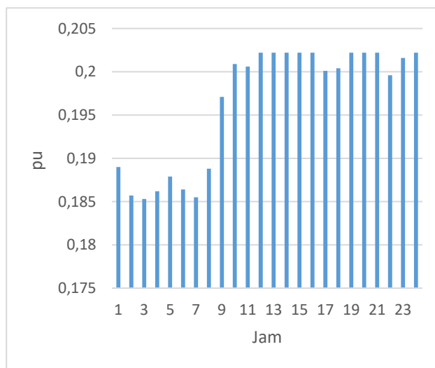
Gbr. 10 Rugi daya aktif setiap jam.
