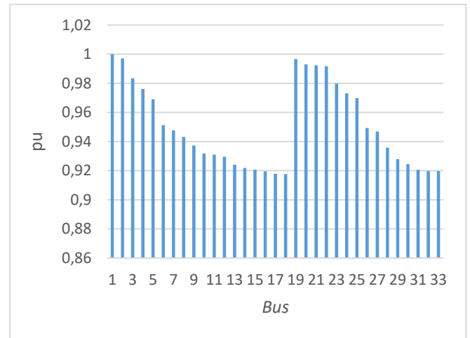
Gbr. 8 Profil tegangan sistem 33 bus IEEE setelah penambahan DG RES.
