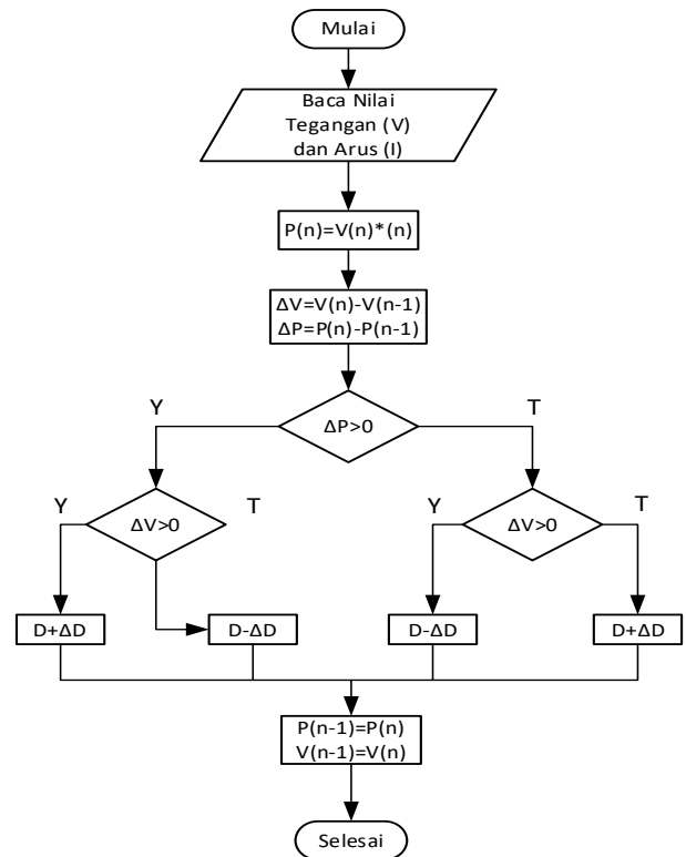
Gambar 3. Prinsip kerja metode P&O.
