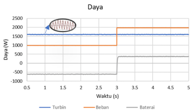
Gambar 8. Daya keluaran turbin angin, daya beban, dan daya baterai ketika kecepatan angin 8 m/s.
