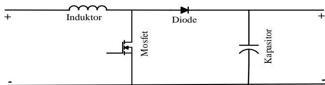
Gambar 2. Rangkaian konverter boost.
