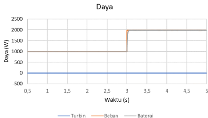
Gambar 11. Daya keluaran turbin angin, daya beban, dan daya baterai ketika kecepatan angin 4 m/s.
