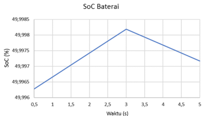
Gambar 10. SoC baterai ketika kecepatan angin 8 m/s.
