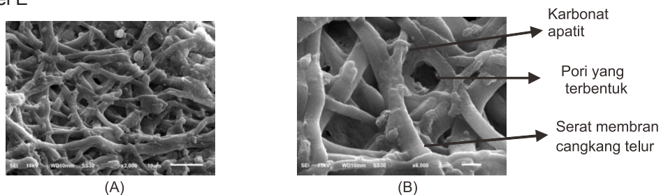
Gambar 5. Hasil karakterisasi SEM Sampel E membran cangkang telur + karbonat apatit + SBF 21 hari (A) perbesaran 2000x dan (B) perbesaran 6000x. Hasil menunjukkan pelepasan apatit lebih banyak dari Sampel D.
