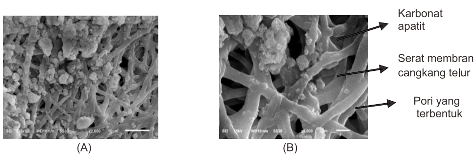
Gambar 3. Hasil karakterisasi SEM Sampel C membran cangkang telur + karbonat apatit + SBF 7 hari (A) perbesaran 2000x dan (B) perbesaran 6000x. Hasil menunjukkan perlekatan apatit pada serat lebih banyak dari Sampel B.
