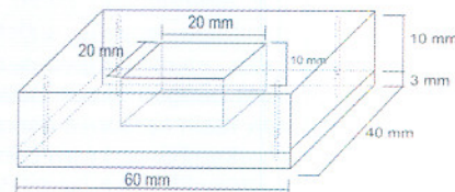
Gambar 2. Cetakan B
