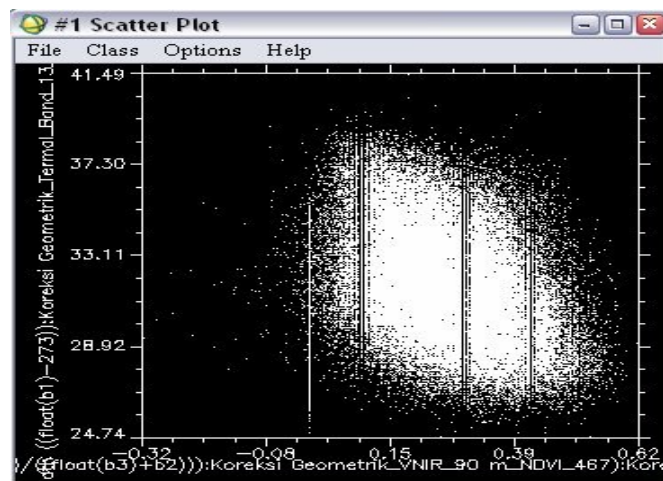
Gambar 1. Scatter Plot indeks TVDI
