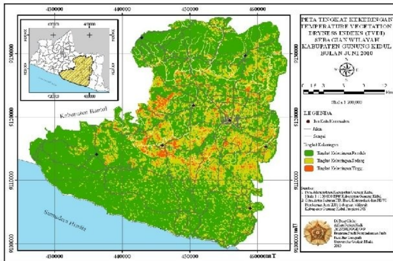
Gambar 3. Peta Tingkat Kekeringan TVDI
