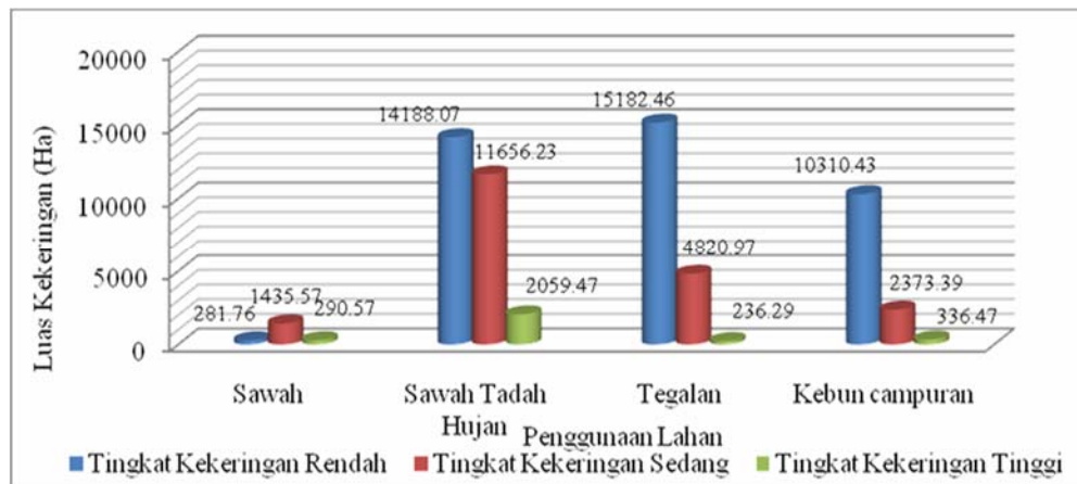
Gambar 5. Luas Kekeringan Berdasarkan Indeks TVDI Berbagai Penggunaan Lahan
