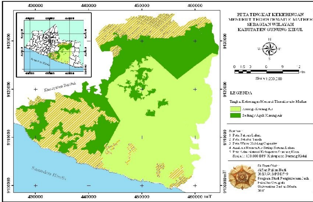
Gambar 6. Peta Tingkat Kekeringan Berdasarkan Klasifikasi Thornthwaite-Mather
