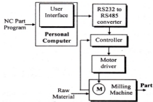
Gambar 4. Hubungan antar komponen sistem CNC retrofit milling
