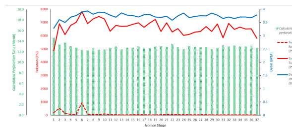
GAMBAR 4. Pengaruh tekanan dan laju alir terhadap waktu perforasi yang dibutuhkan.
