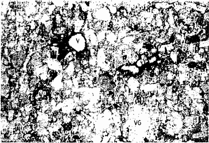
Figure 1. Struktur mikro intergrain dan pellicular grain pada hor.B31g pedon Mer-I. Plane-polarisasi 30x.
