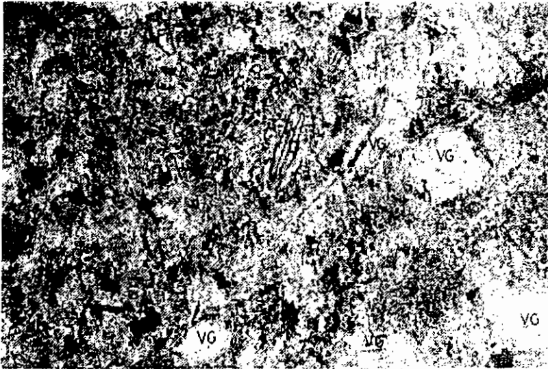
Figure 4. Diatom (D), fitolit (opaline silica) dan glas volkan (VG) pada matrix hor.Aplg pedon Mer-6. Plane-polarisasi 30x.
