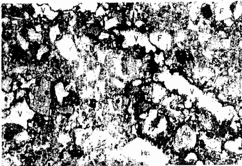
Figure 6. Nodule dan coating Fe-hidroksida dijumpai tersebar pada hor.B3gm pedon Mer-3. Komposisi mineral, augit (Ag), hornblende (Hn), felspar (F), pumis (P). Pl-polarisasi 30x.
