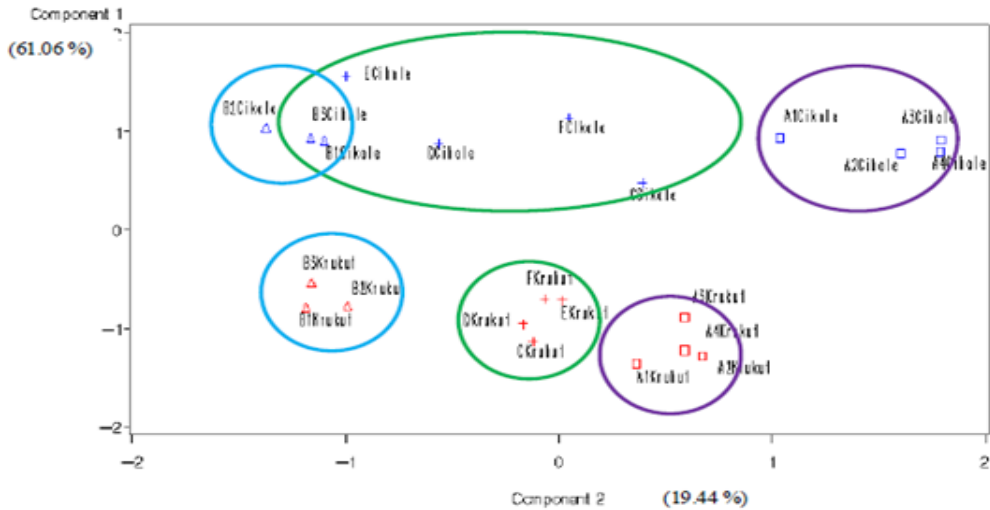
Gambar 2. Diagram Pancar Analisis Komponen Utama
