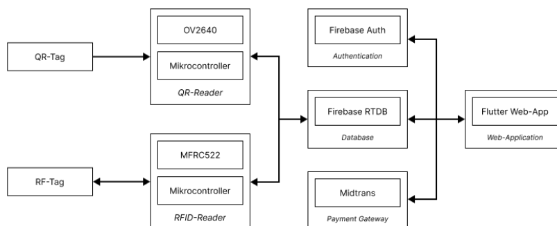
Gambar 2.2 Diagram Arsitektur Sistem
