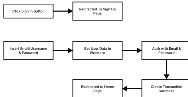
Gambar 2.6 Diagram Proses pada Sign-in Page
