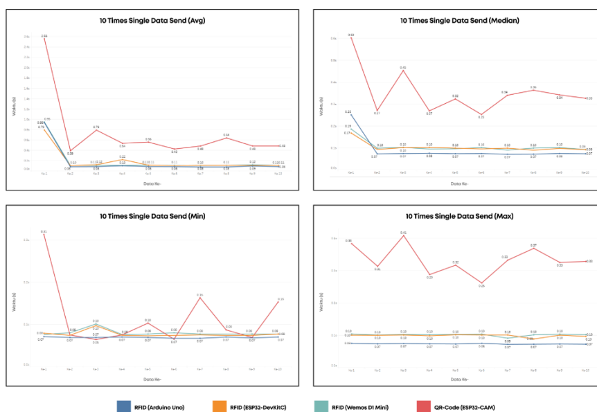
Gambar 3.3 Hasil Pengujian Pembacaan dan Pengiriman Data Barang Statis ke Firebase
