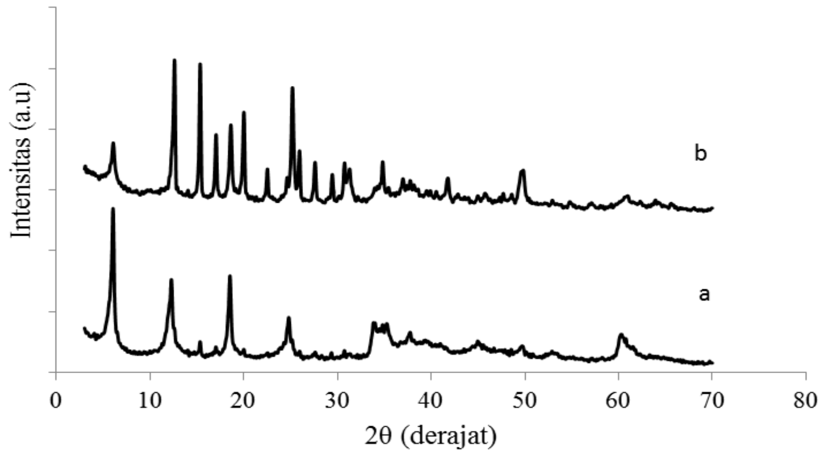
Gambar 5. Difraktogram padatan hidrotalsit Zn-Al-EDTA; (a) sebelum desorpsi dan (b) sesudah desorpsi.
