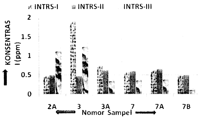
Gambar 6. Grafik Pengaruh Lubang Resapan Biopori Terhadap Tingkat Intrusi Air Laut dalam Air Sumur Gali Daerah Penelitian
