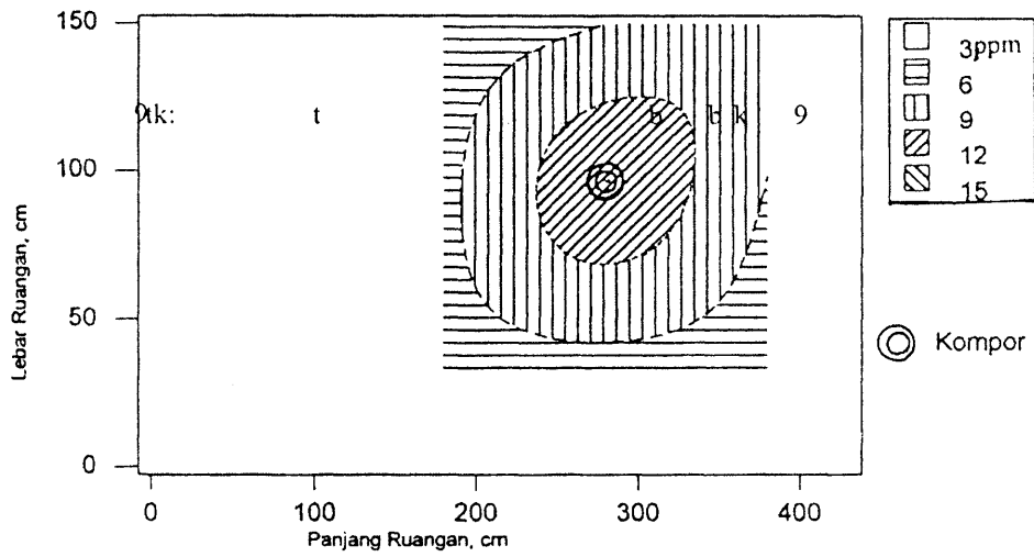
Gambar 9. Pandangan Atas Sebaran CO di Ruang Proses Pematikan Industri T pada Ketinggian 160 cm
