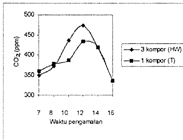
Gambar 2. Konsentrasi CO 2 di Ruang Proses Pematikan Industri HW dan Industri T.
