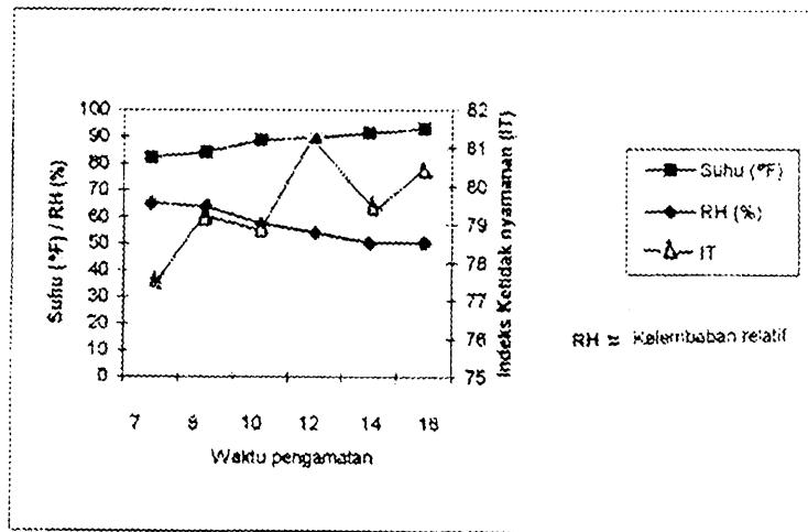
Gambar 6. Indeks Ketidaknyamanan di Ruang Proses Pematikan HW
