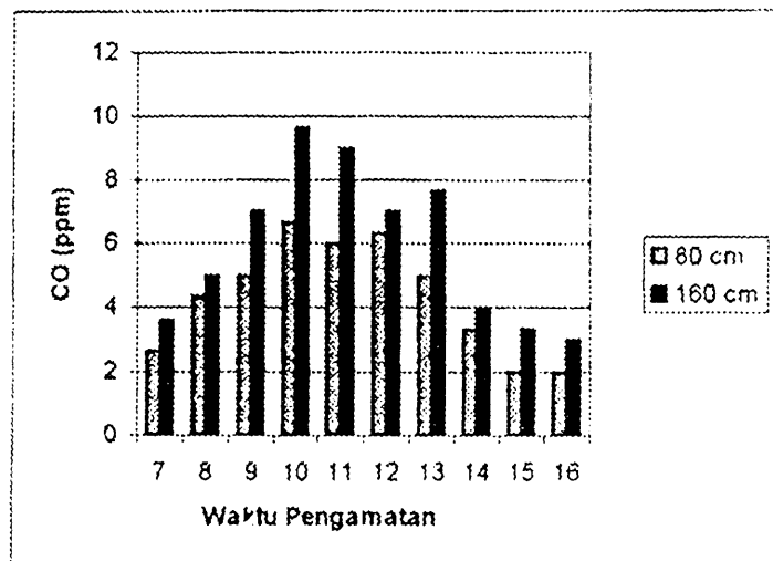
Gambar 11. Konsentrasi CO di Ruang Proses Pematikan Industri T pada Ketinggian 80 cm dan 160 cm pada Kordinat (280,90) dari Sudut Ruangan (0,0) Pandangan Atas.
