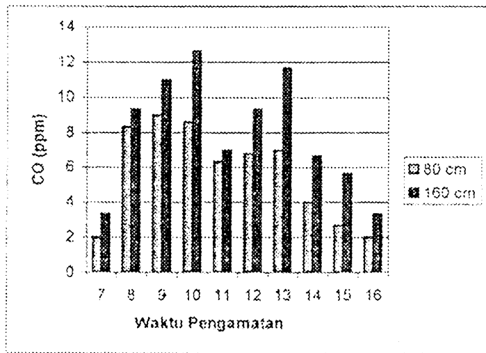
Gambar 10. Konsentrasi CO di Ruang Proses Pematikan Industri HW pada Ketinggian 80 cm dan 160 cm pada Kordinat (150,90) dari Sudut Ruangan (0,0) Pandangan Atas.
